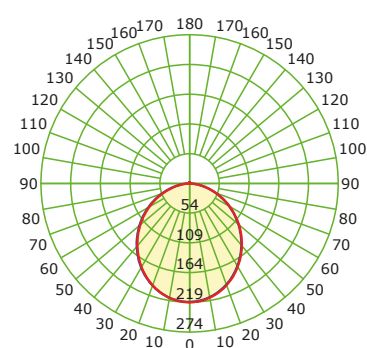
CURVA FOTOMETRICA
